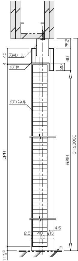
縦断面図
