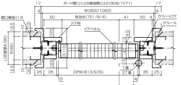
横断面図
