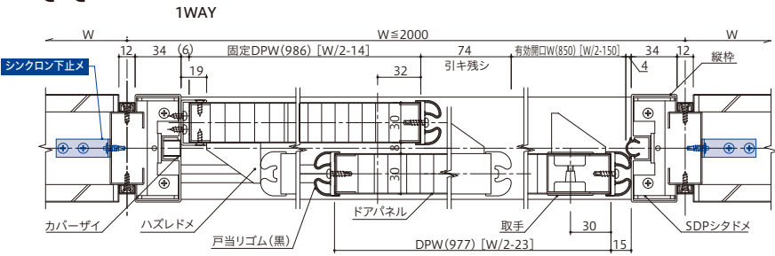
C-C
