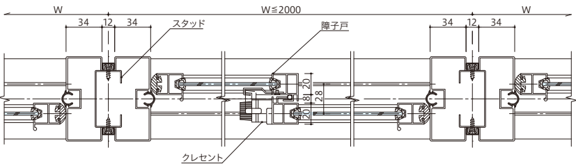
B-B
