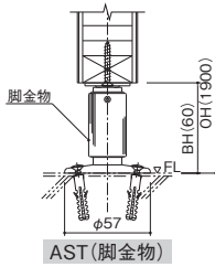
AST(脚金物)
